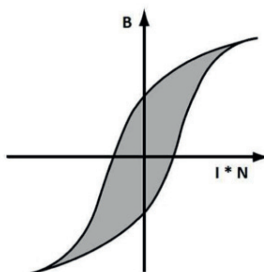
Fig. 1 Cycle d'hystérésis [3]
