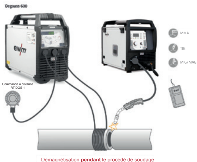
Fig. 8 Représentation schématique : Génération d'un champ magnétique opposé pendant le soudage
